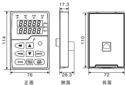
键盘尺寸图
