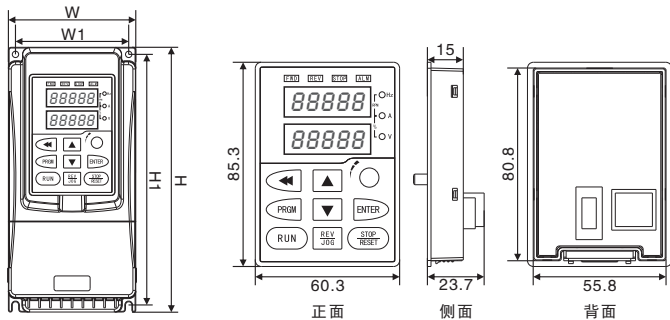
键盘托尺寸图
