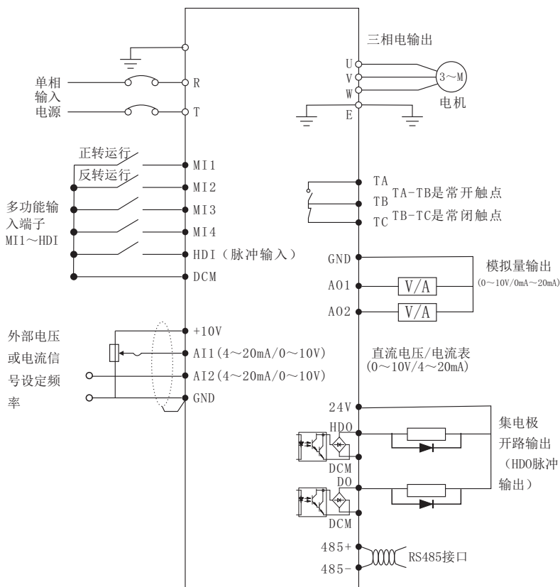
S款 单相0.75~2.2kw标准配线图
