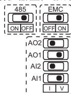
N款 0.75kW-7.5kW主控板开关设置
