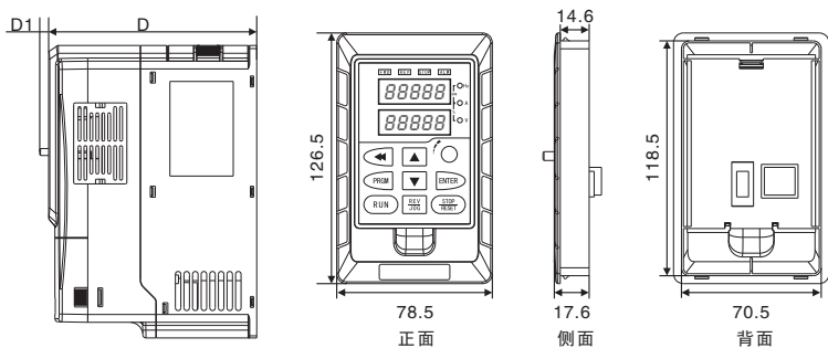
S款 0.75~7.5KW系列机箱规格表
