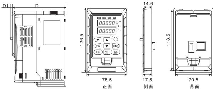
N款 0.75-7.5KW系列机箱规格表
